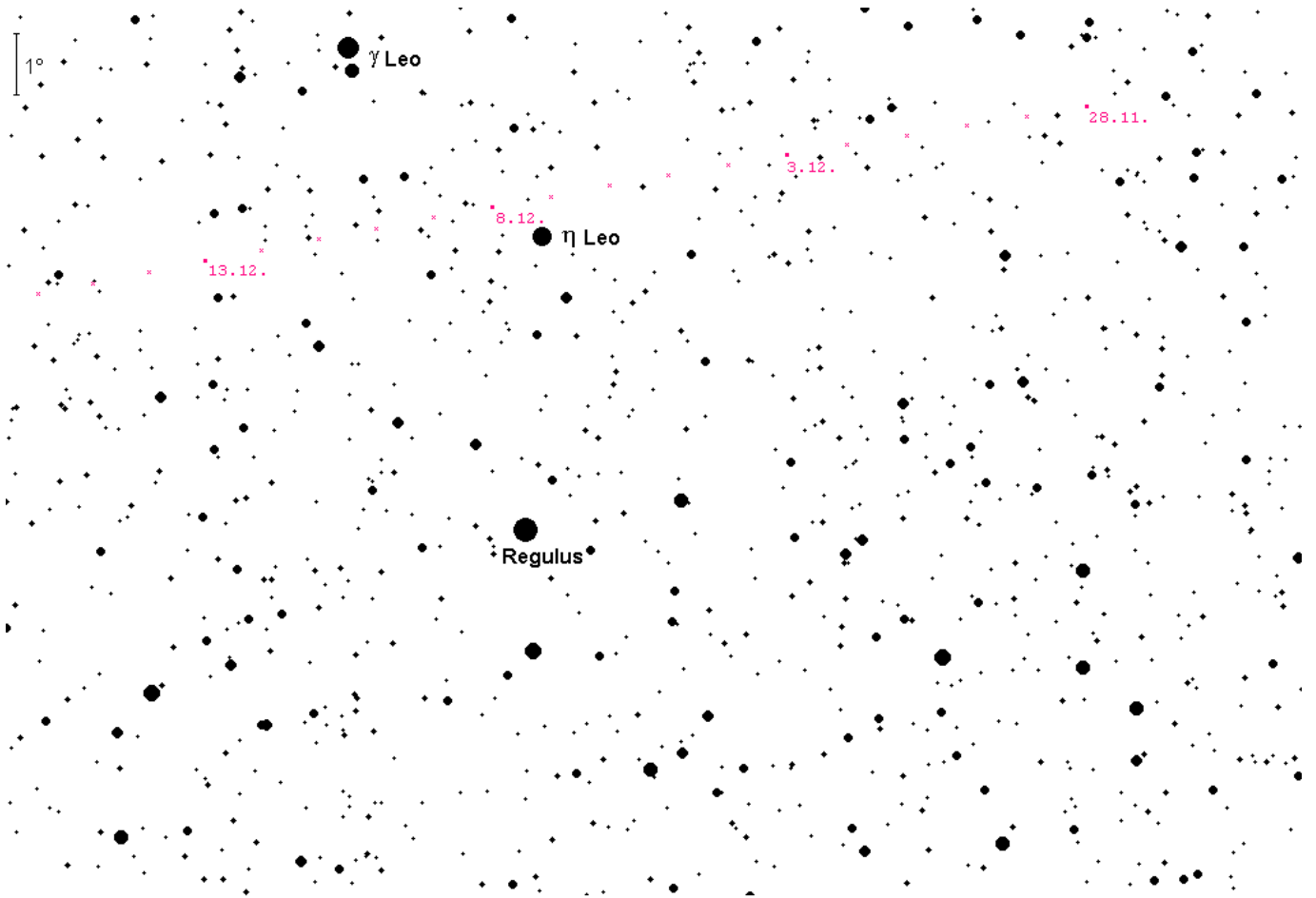
Bewegung des Kometen 62P/Tsuchinshan vom 28.11.2023 bis 16.12.2023
