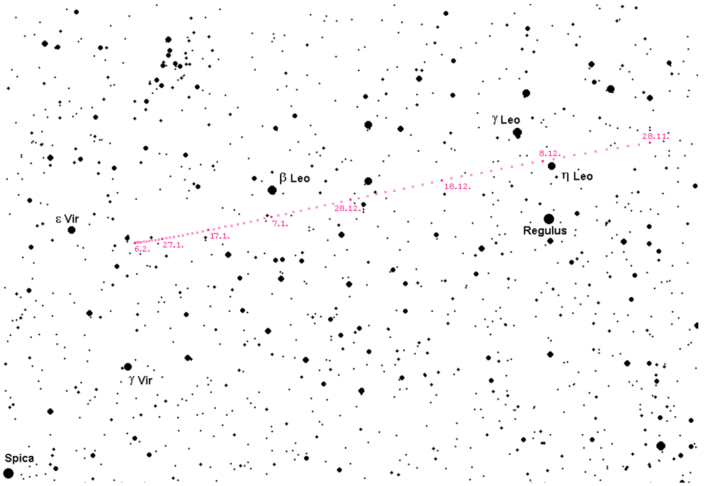
Bewegung des Kometen 62P/Tsuchinshan vom 28.11.2023 bis 6.2.2024
