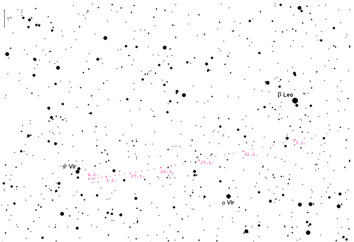
Bewegung des Kometen 62P/Tsuchinshan vom 2.1.2024 bis 6.2.2024
