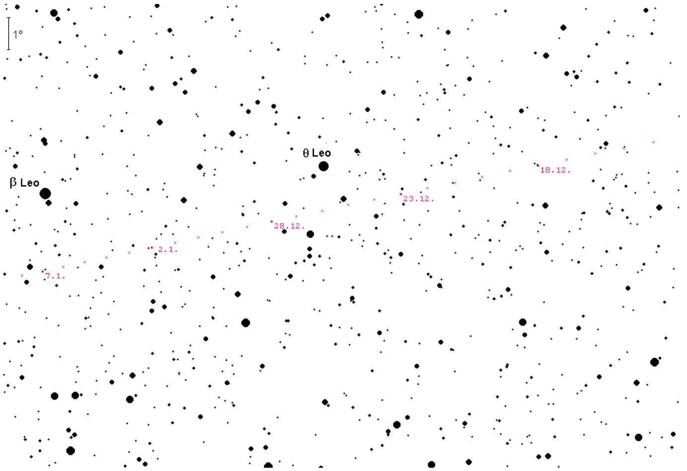
Bewegung des Kometen 62P/Tsuchinshan vom 14.12.2023 bis 8.1.2024
