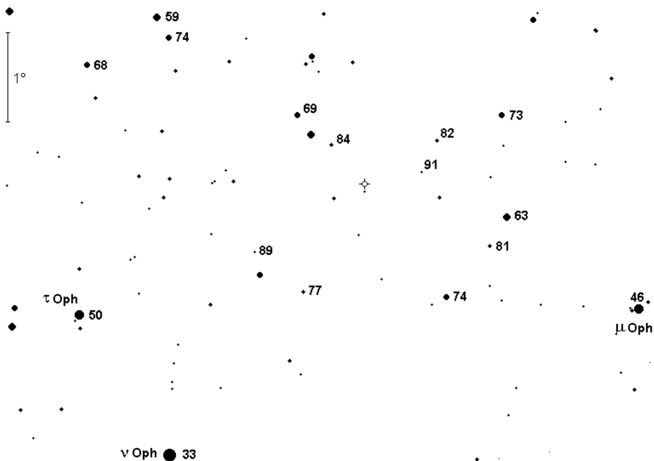
Vergleichssternkarte für die rekurrierende Nova RS Ophiuchi
