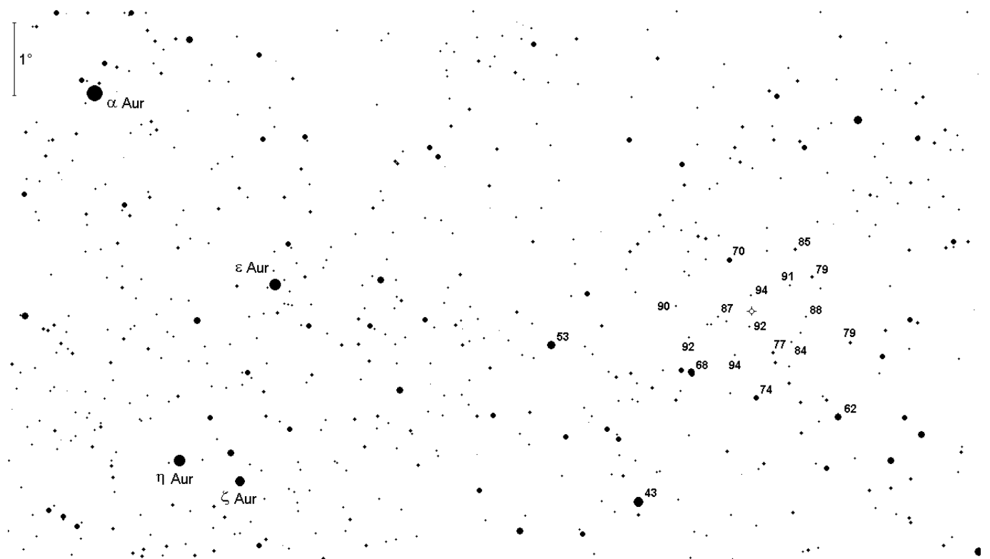
Vergleichssternkarte für die Nova Persei 2020
